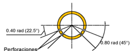
Corte transversal
