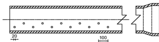
Corte longitudinal
